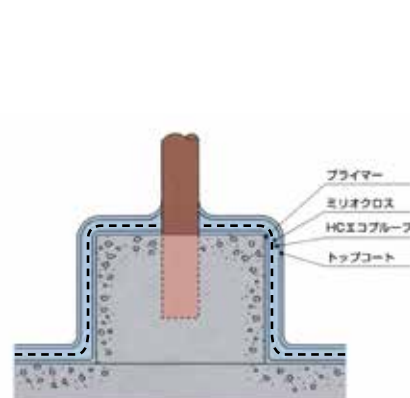
基礎廻り
