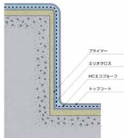
立面部(1)
