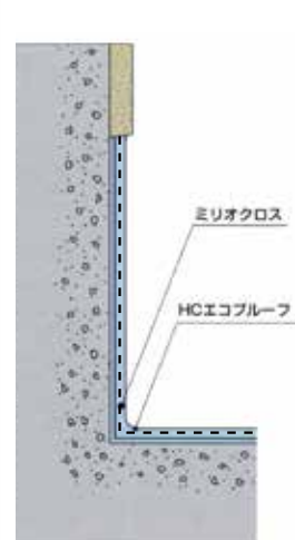
立面部(2)
