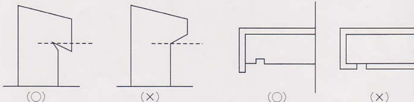
(軒先部)
