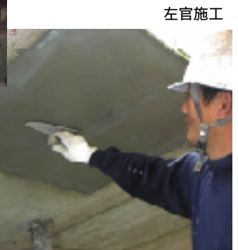
左官施工
